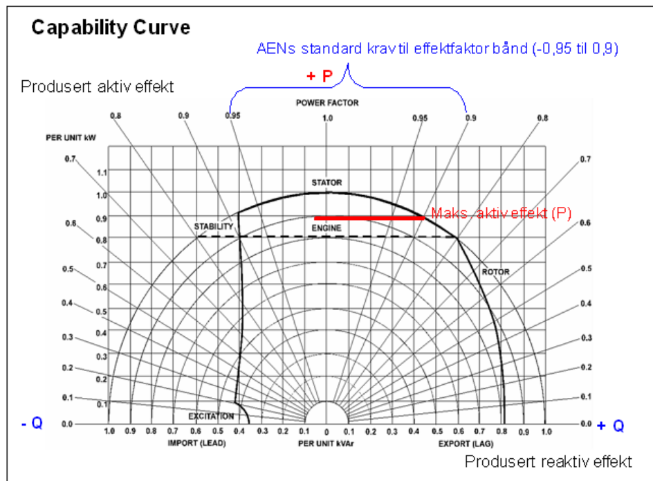
Figur 2 Eksempel på driftsdiagram ("Capability Curve") for synkrongenerator.
